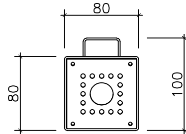
PLANTA TopView
